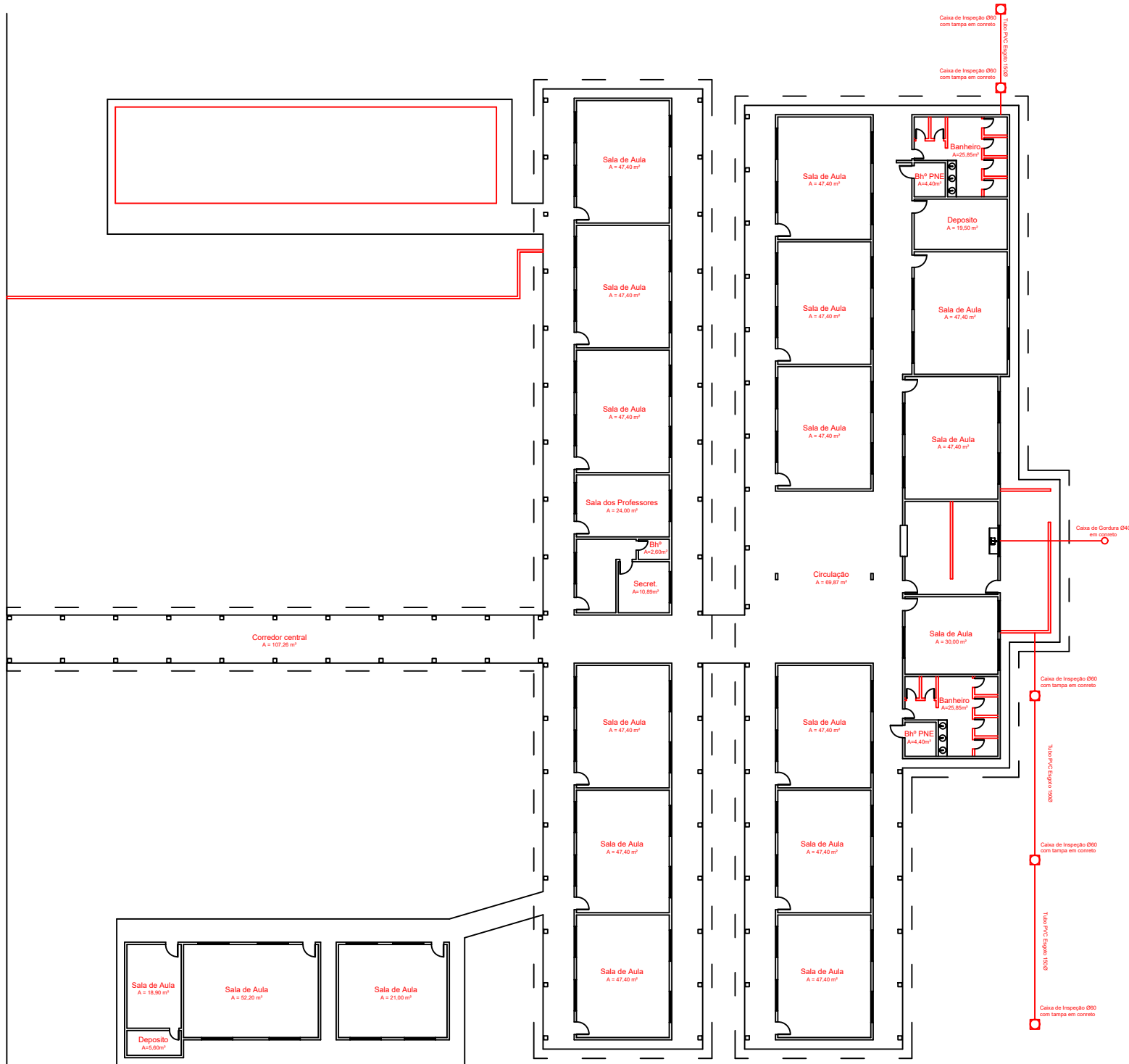
Planta Baixa Esc. 1 / 125
