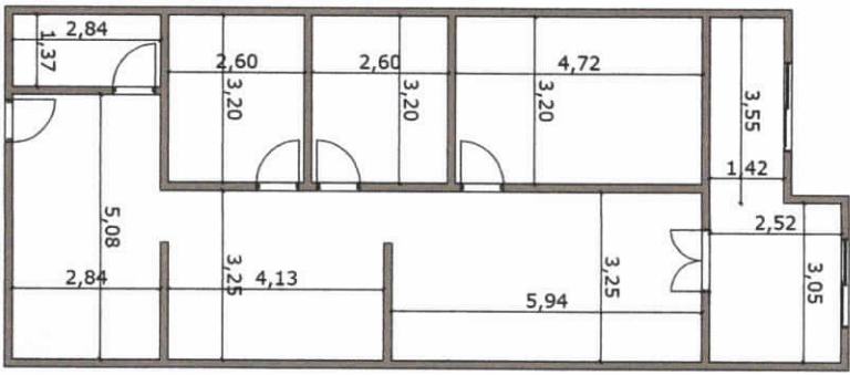
1 TÉRREO 1:50
