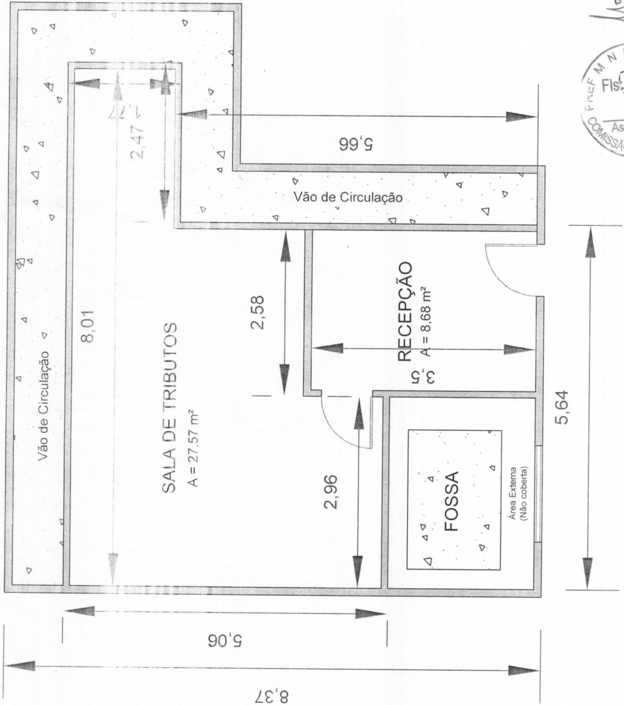
PLANTA BAIXA
