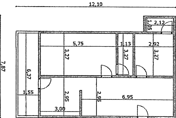
1 TERREO 1:50
